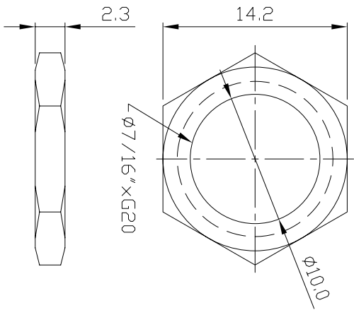
NUT
