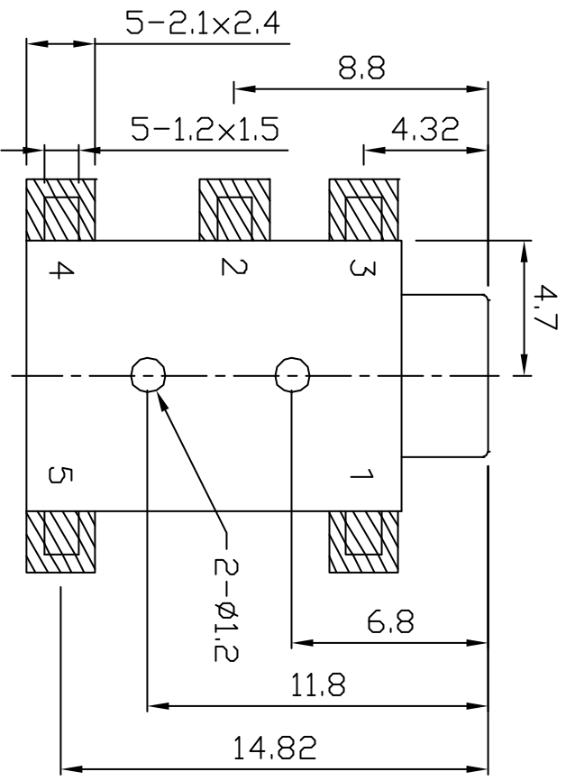
PLUG P.C.B. LAYOUT(±0.1) BOTTOM VIEW
