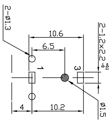
P.C.B LAYOUT(±0.1) (BOTTOM VIEW)
