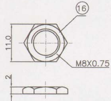
NUT 1PC
